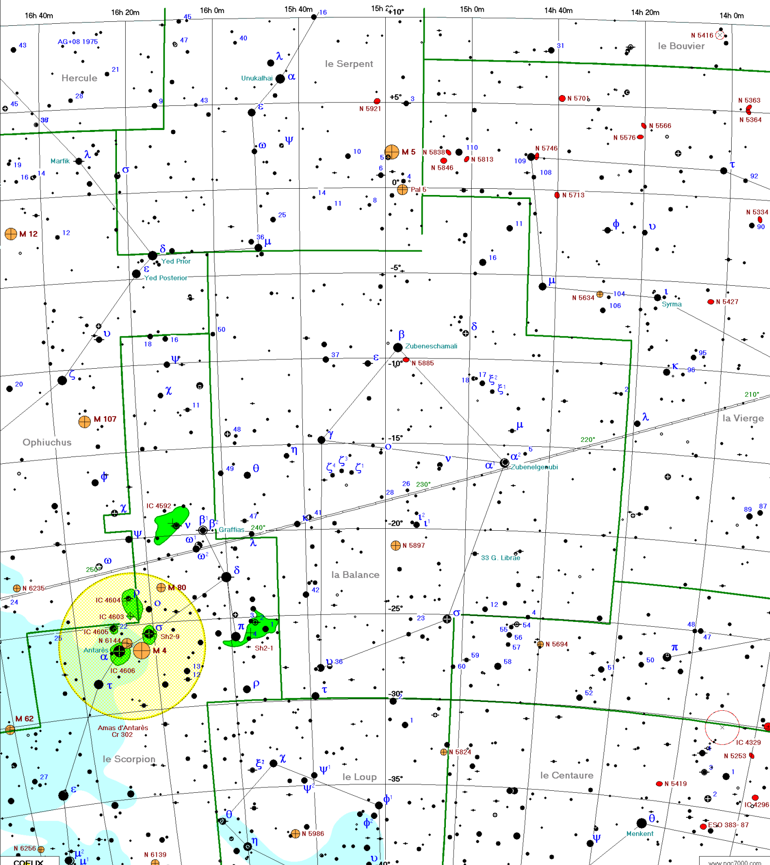
Magnitudes stellaires
