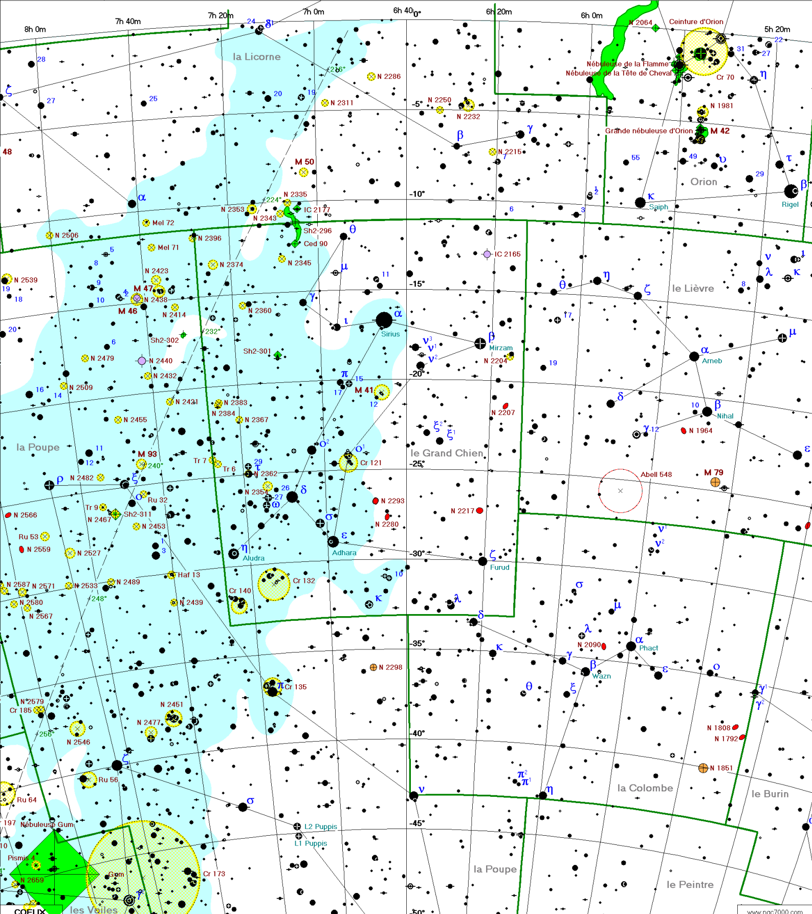
Magnitudes stellaires
