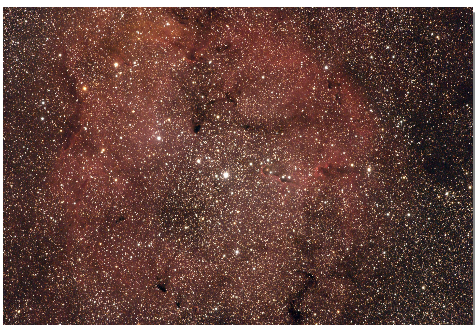
IC 1396 (Céphée)
