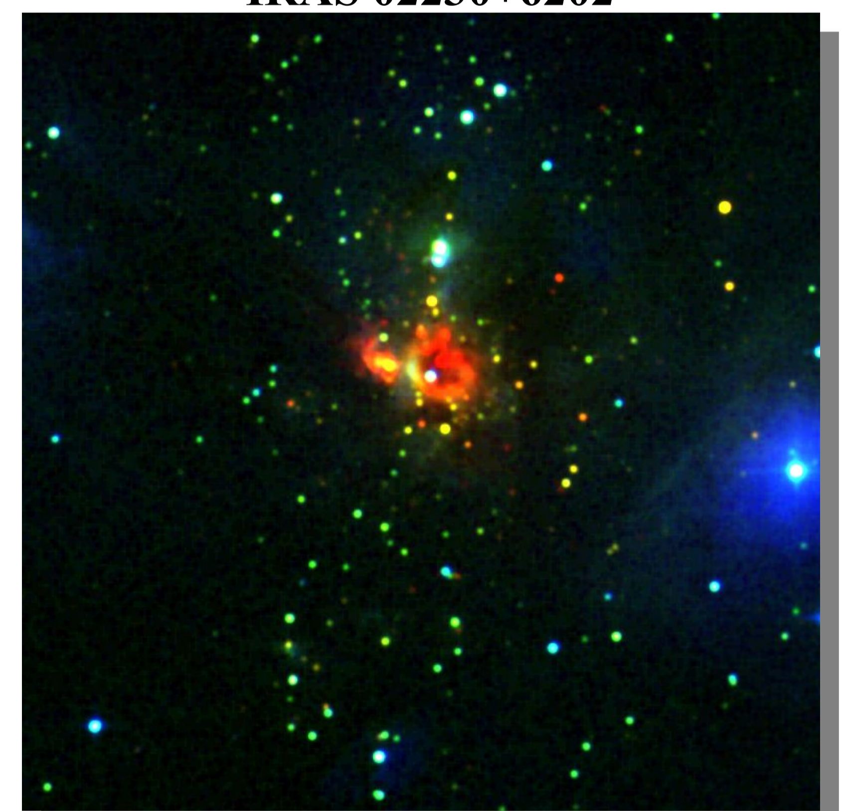
IRAS 06053-0622
