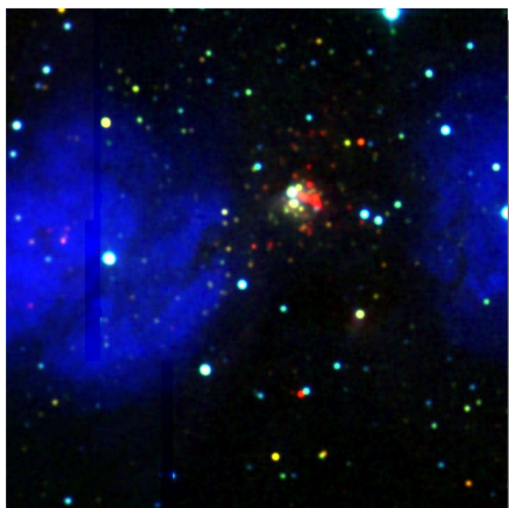
IRAS 06099+1800
