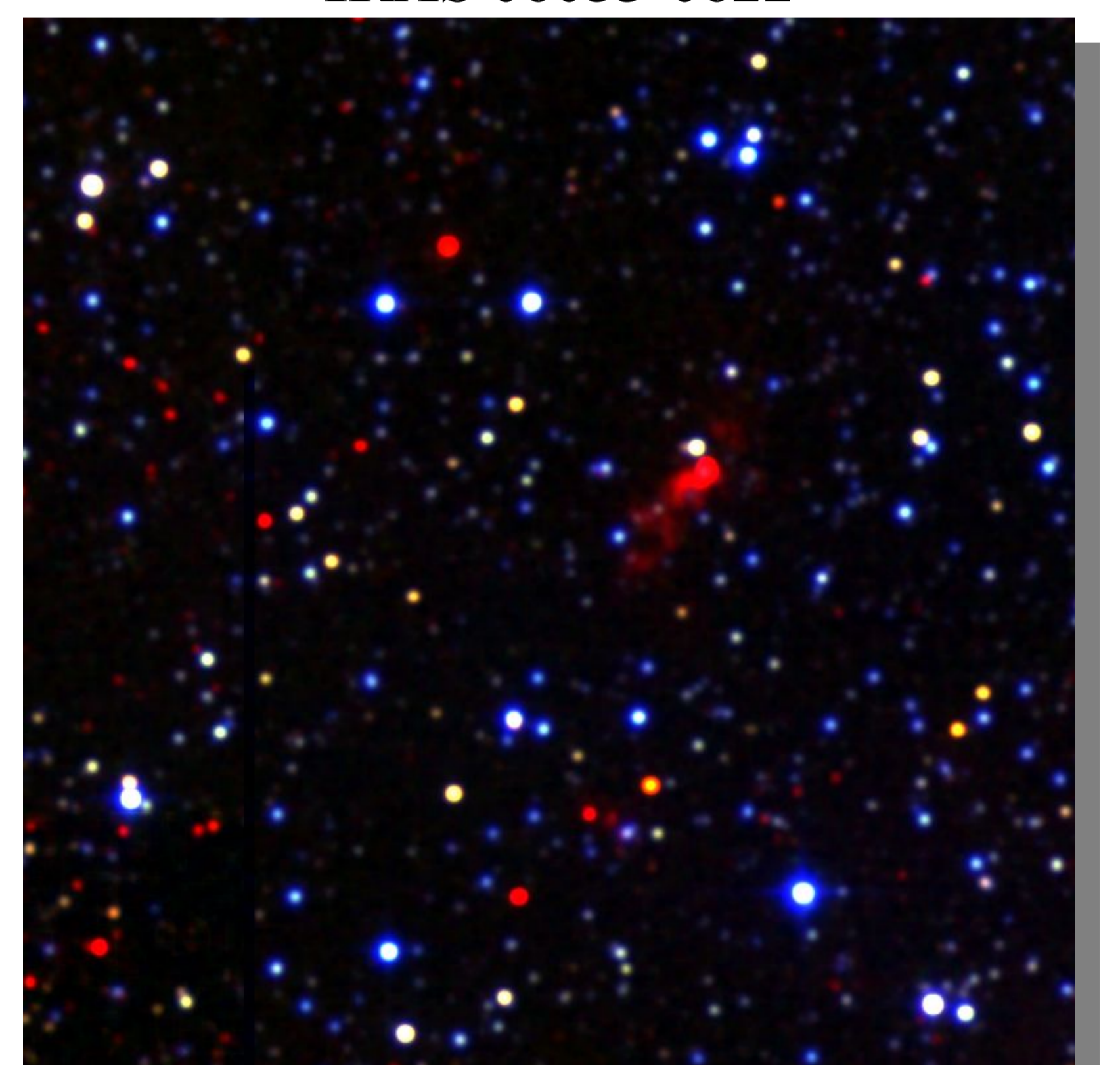
IRAS 18117-1753
