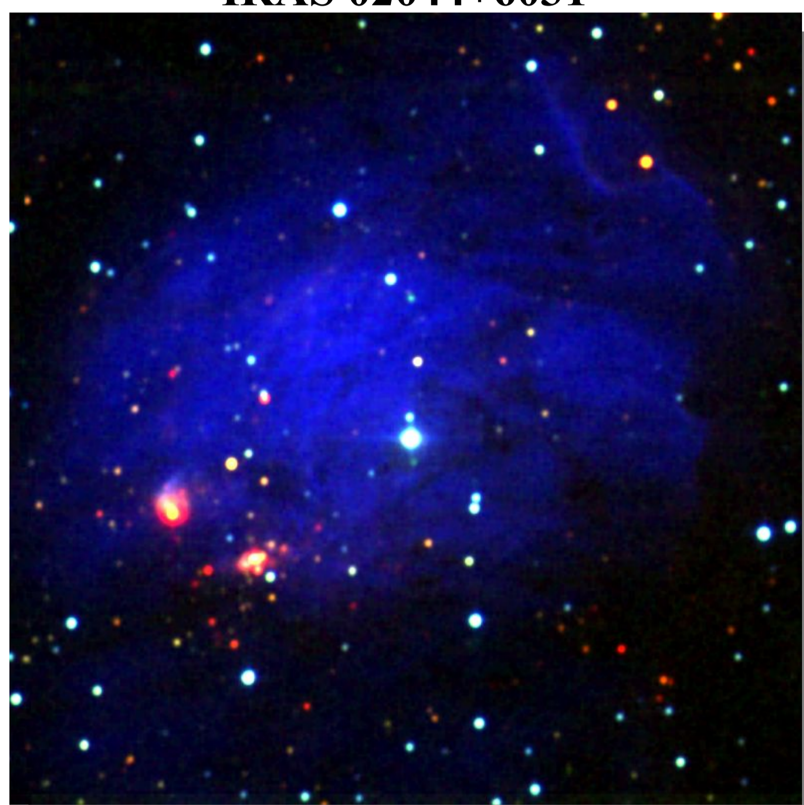
IRAS 05374+3549
